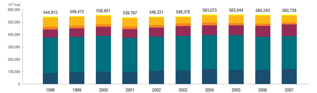
Primary energy supply (Japan) 一次エネルギー供給実績 (国内)
